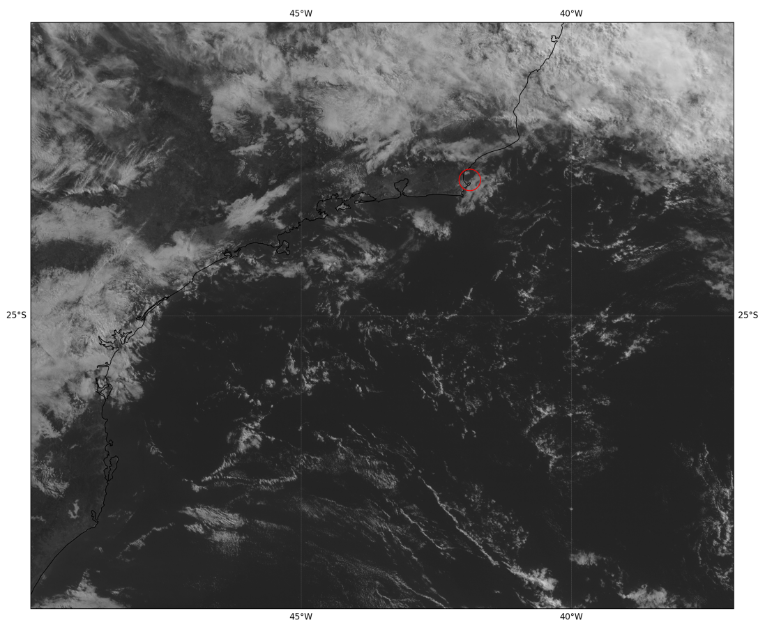
Imagem do satélite GOES-19 - Canal Visível do dia 2025-04-15 11:50 UTC
