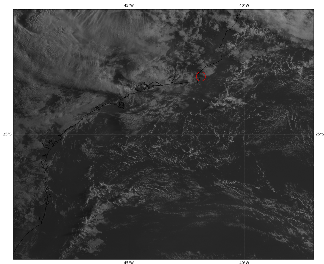
Imagem do satélite GOES-19 - Canal Visível do dia 2025-04-18 10:00 UTC
